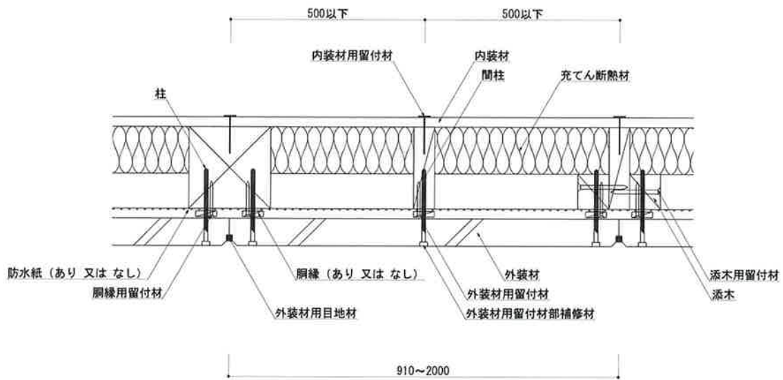
図2 構造説明図 (断面図・外壁ヨコ張り／構造用面材なし／内装材／充填断熱材あり)
