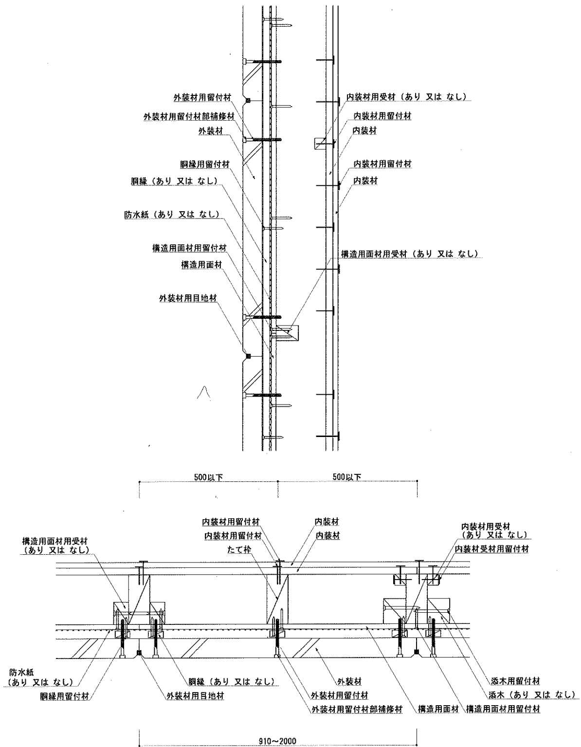
断面図(内装材(重張)・充てん断熱材なし)
