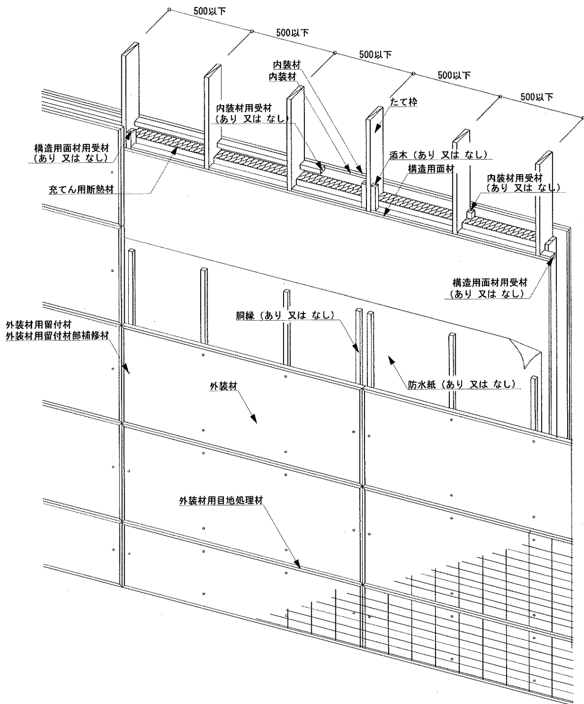
透視図(内装材(重張)・充てん断熱材あり)
