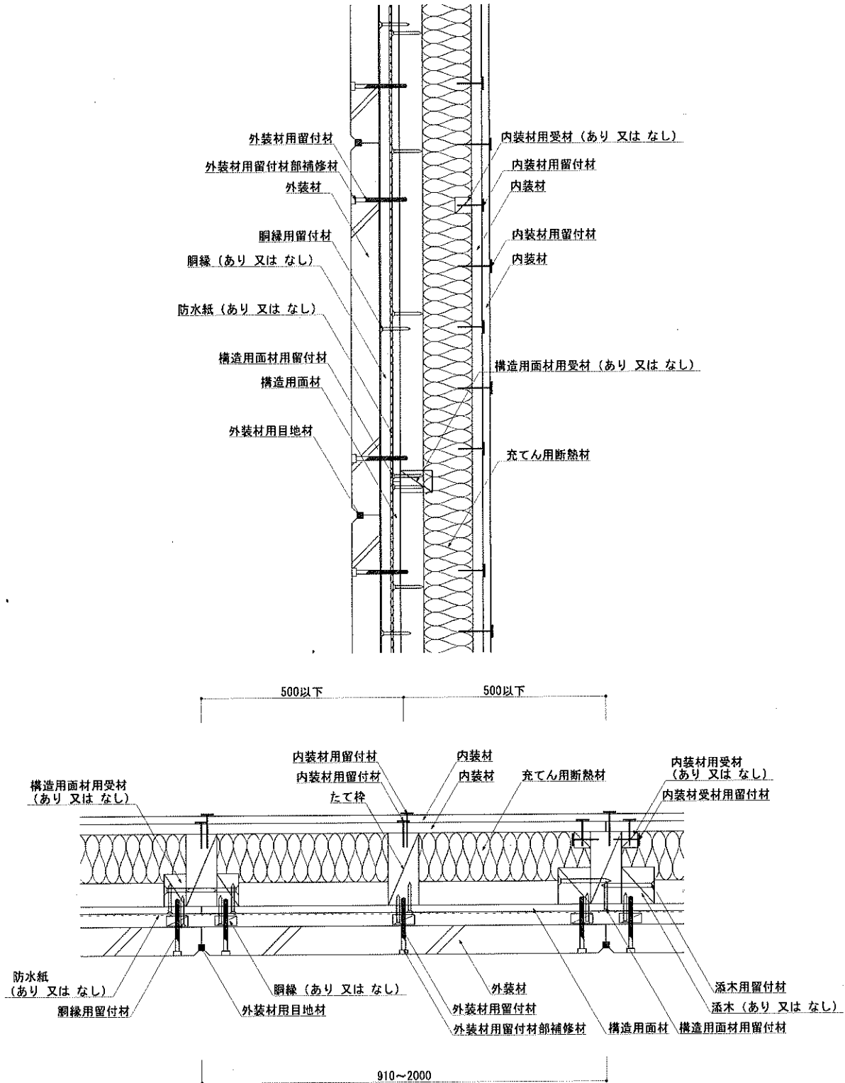
断面図(内装材(重張)・充てん断熱材あり)
