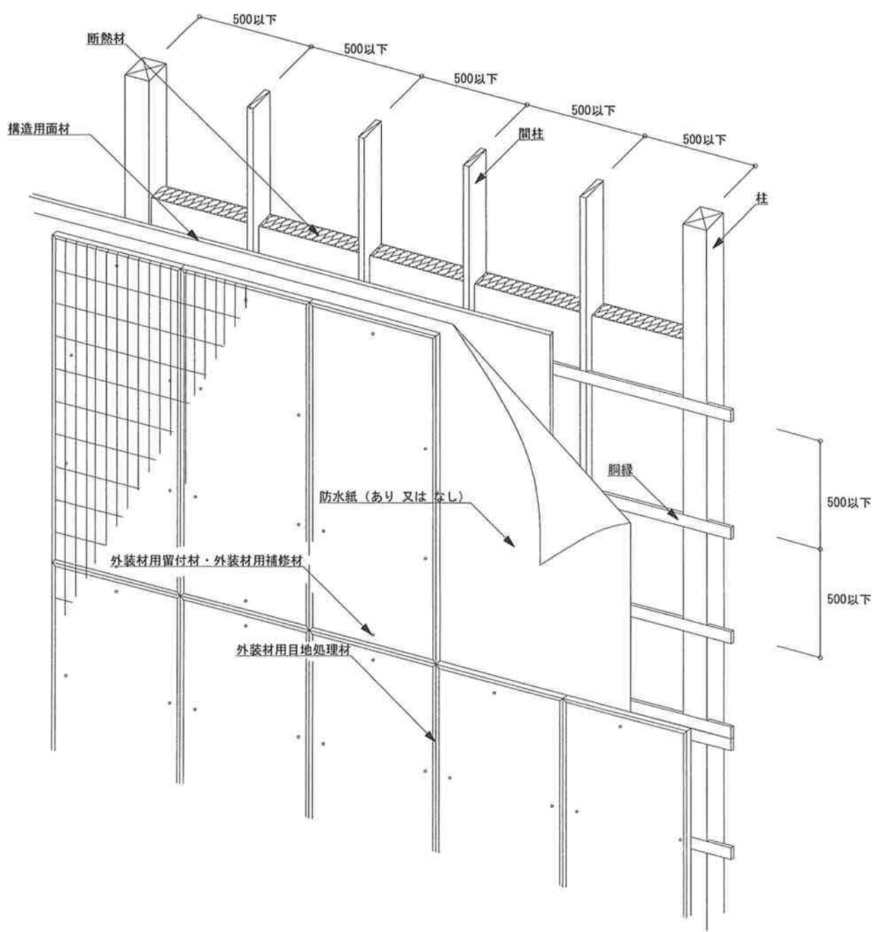
図3 構造説明図 (透視図・胴縁取付仕様2・構造用面材あり・断熱材あり)
