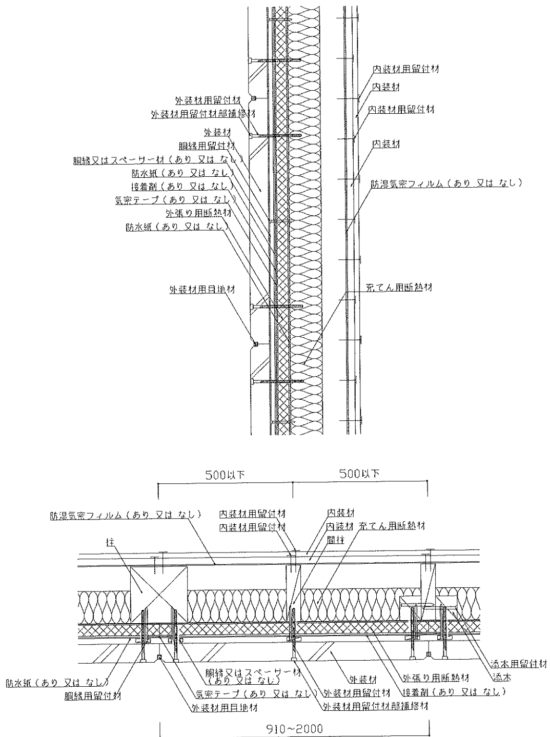
図2 構造説明図 (断面図・構造用面材なし/内装材大壁(重張)/充てん用断熱材あり)
