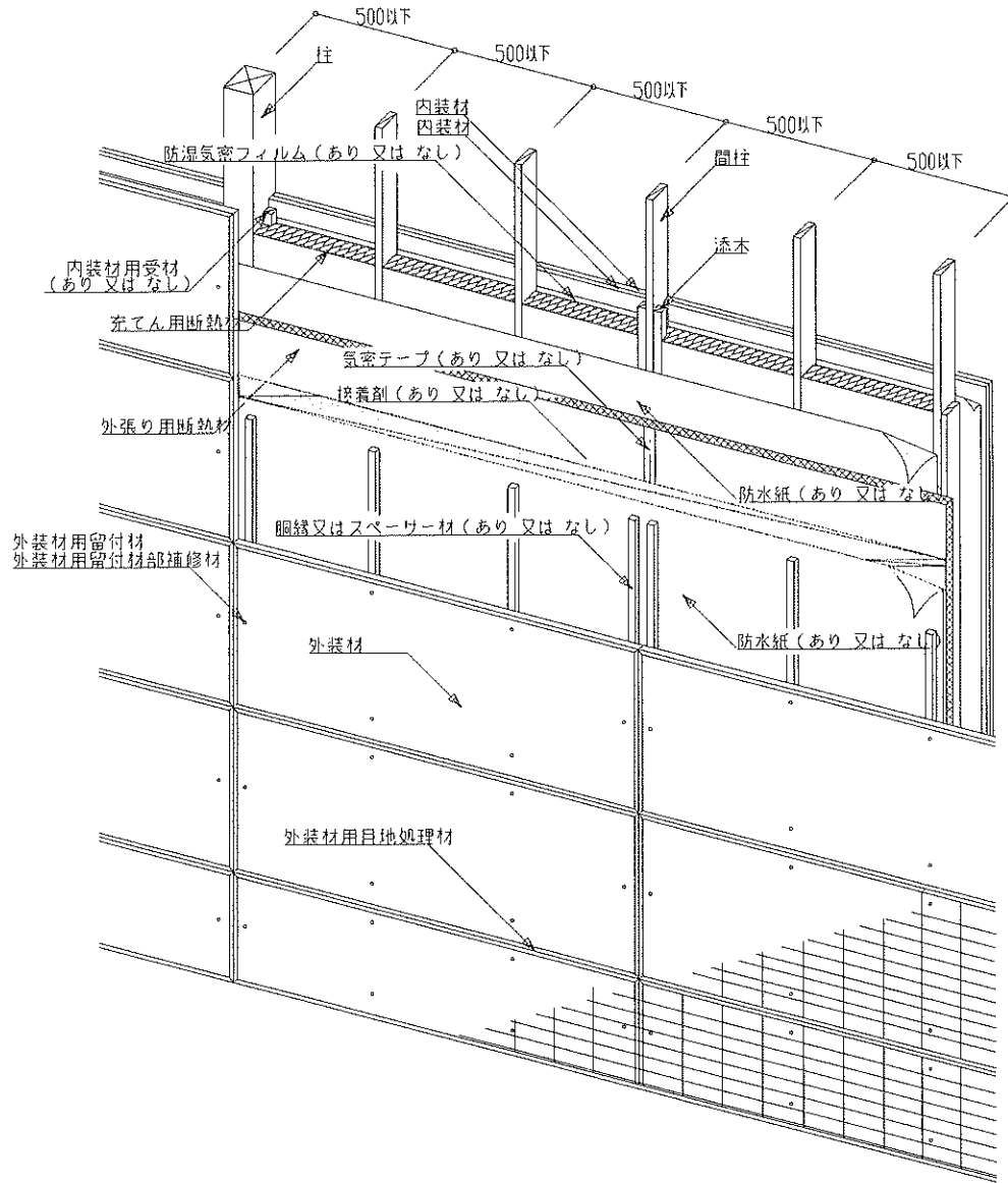
図3 構造説明図 (透視図・構造用面材なし／内装材真壁(重張)／充てん用断熱材あり)
