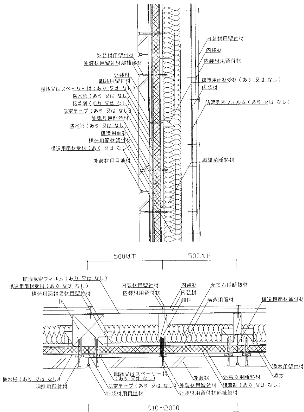
図6 構造説明図 (断面図・構造用面材真壁/内装材大壁(重張)/充てん用断熱材あり)
