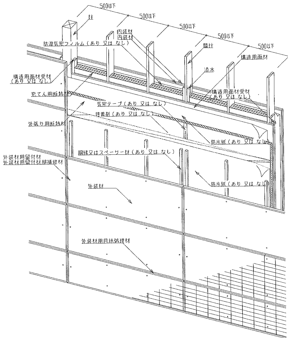
図5 構造説明図 (透視図・構造用面材真壁／内装材大壁(重張)／充てん用断熱材あり)
