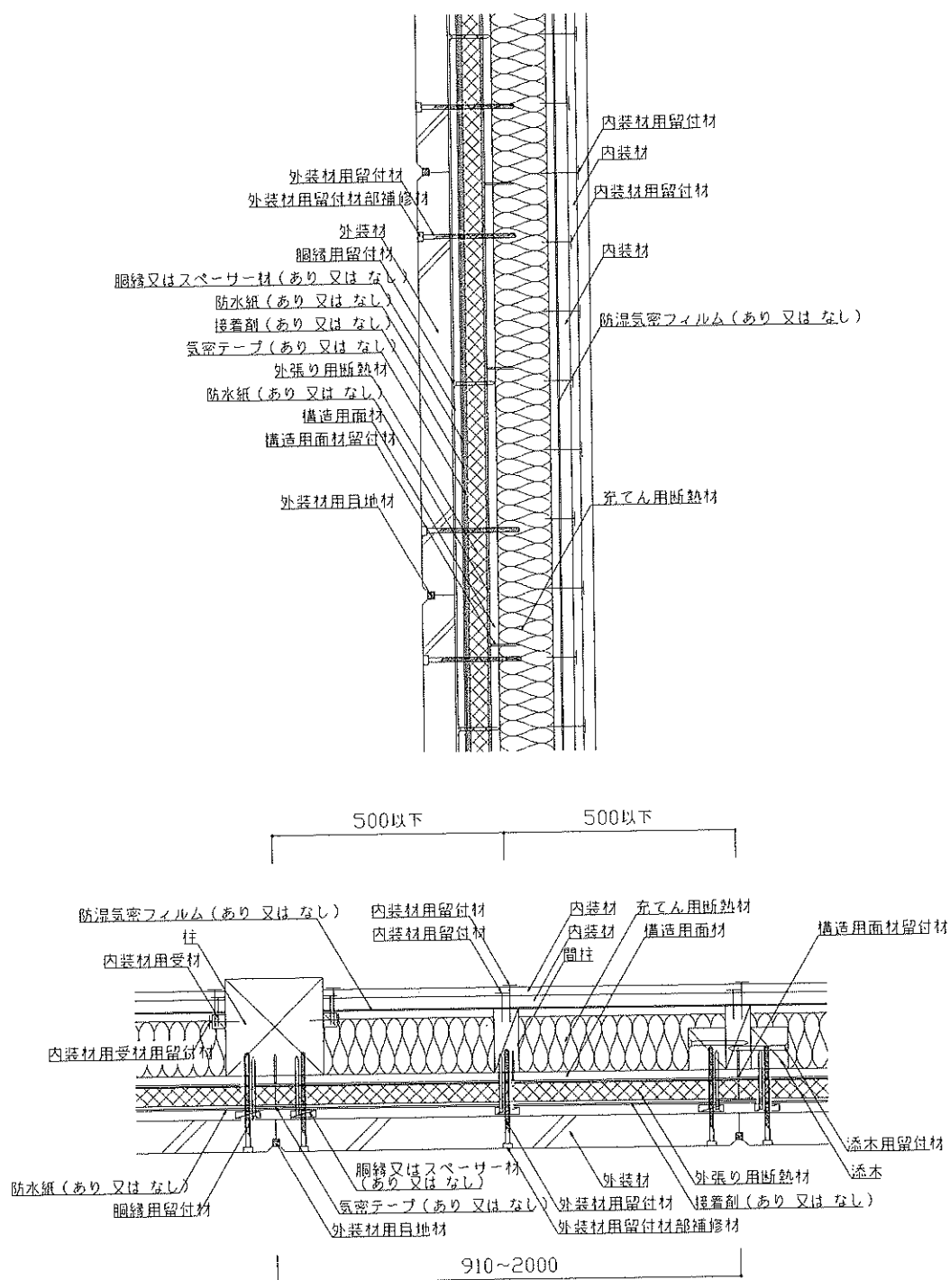
図4 構造説明図 (断面図・構造用面材大壁／内装材真壁(重張)／充填用断熱材あり)
