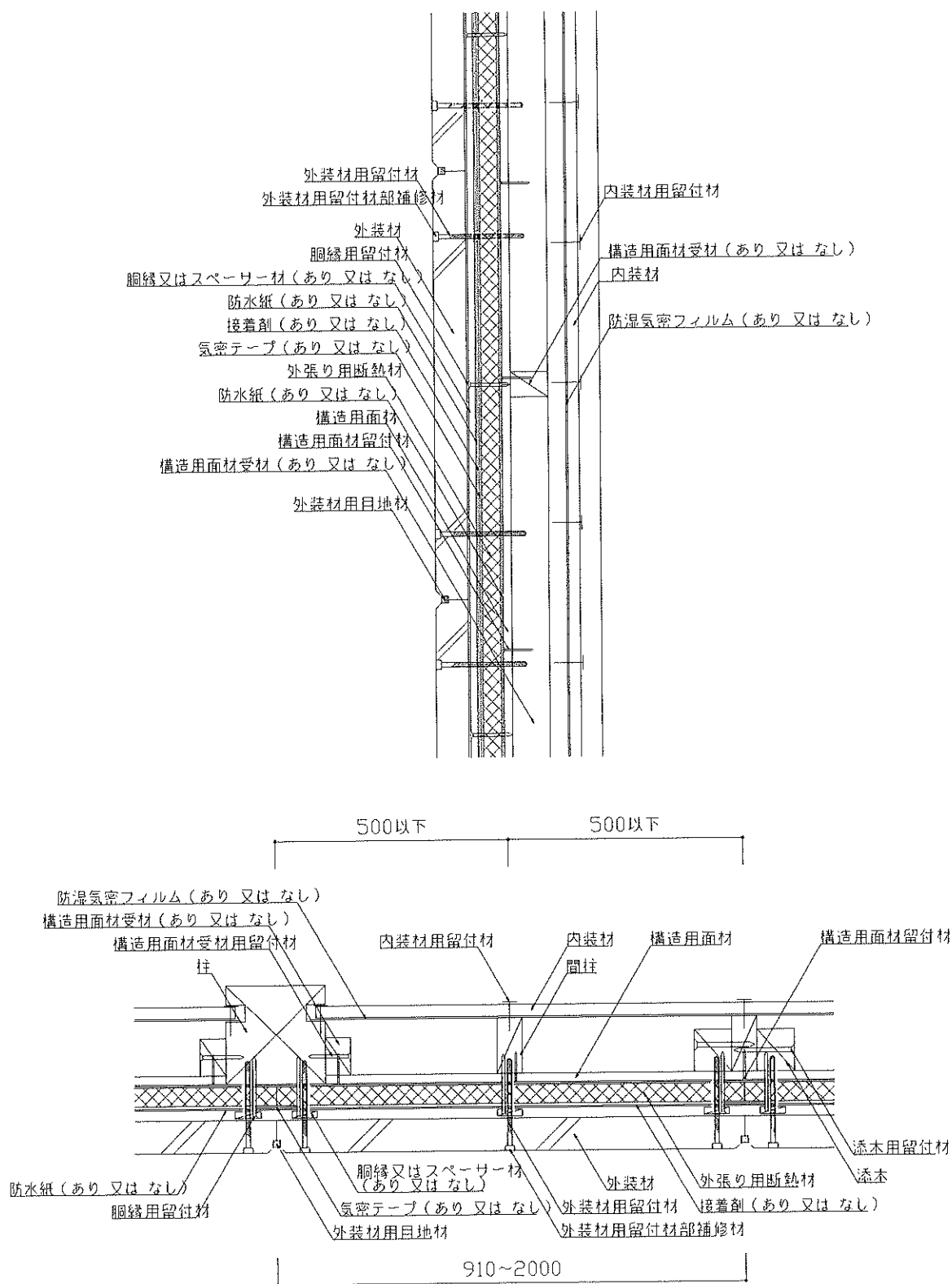
図8 構造説明図 (断面図・構造用面材真壁／内装材真壁(単張①)／充てん用断熱材なし)
