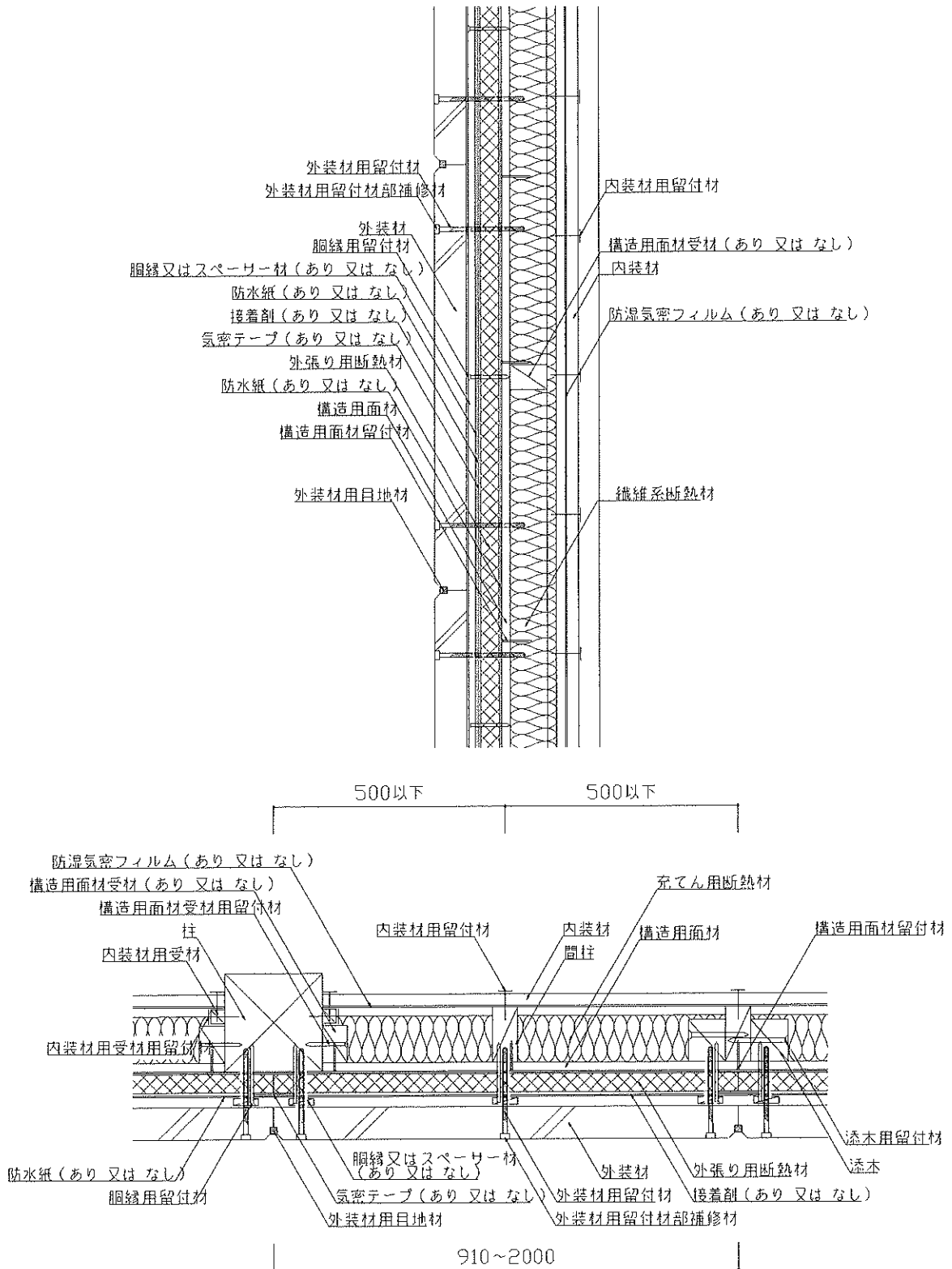
図12 構造説明図 (断面図・構造用面材真壁/内装材真壁(単張②)/充てん用断熱材あり)
