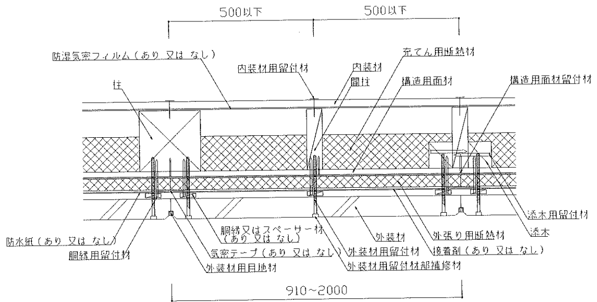
図2 構造説明図 (断面図・構造用面材大壁／内装材大壁(単張))
