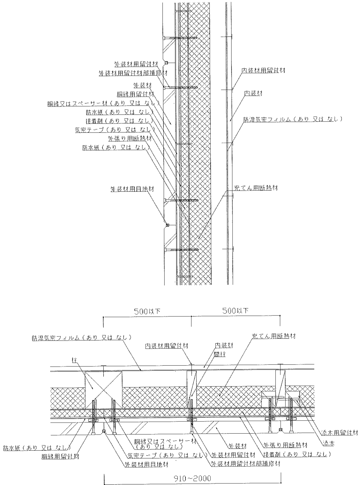
図2 構造説明図 (断面図・構造用面材なし/内装材大壁(単張))
