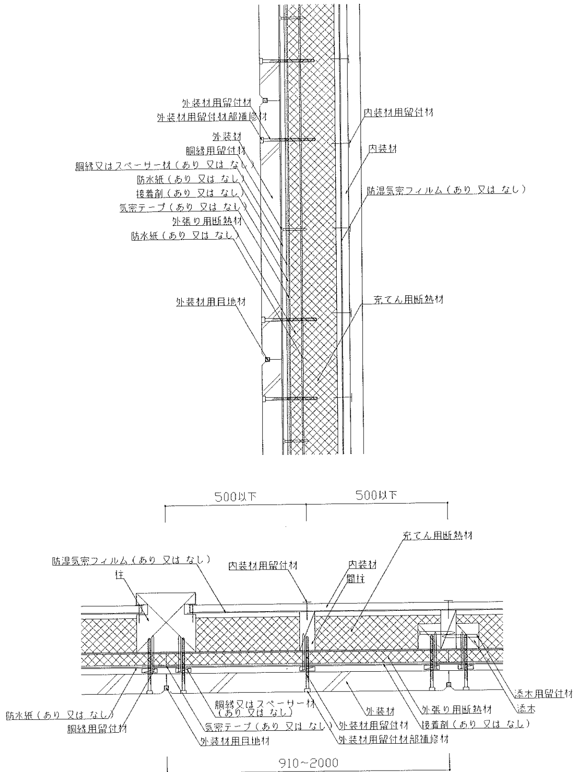
図4 構造説明図 (断面図・構造用面材なし/内装材真壁(単張①))
