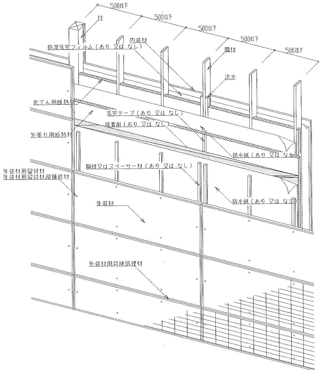
図3 構造説明図 (透視図・構造用面材なし/内装材真壁(単張①))
