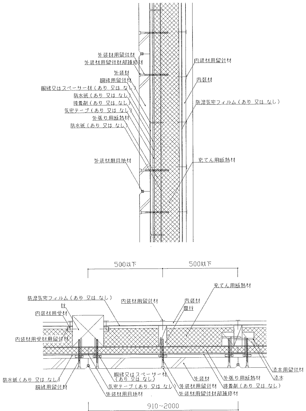
図6 構造説明図 (断面図・構造用面材なし/内装材真壁(単張②))
