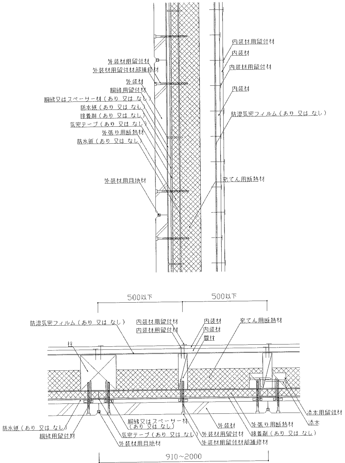
図2 構造説明図 (断面図・構造用面材なし/内装材大壁(重張))
