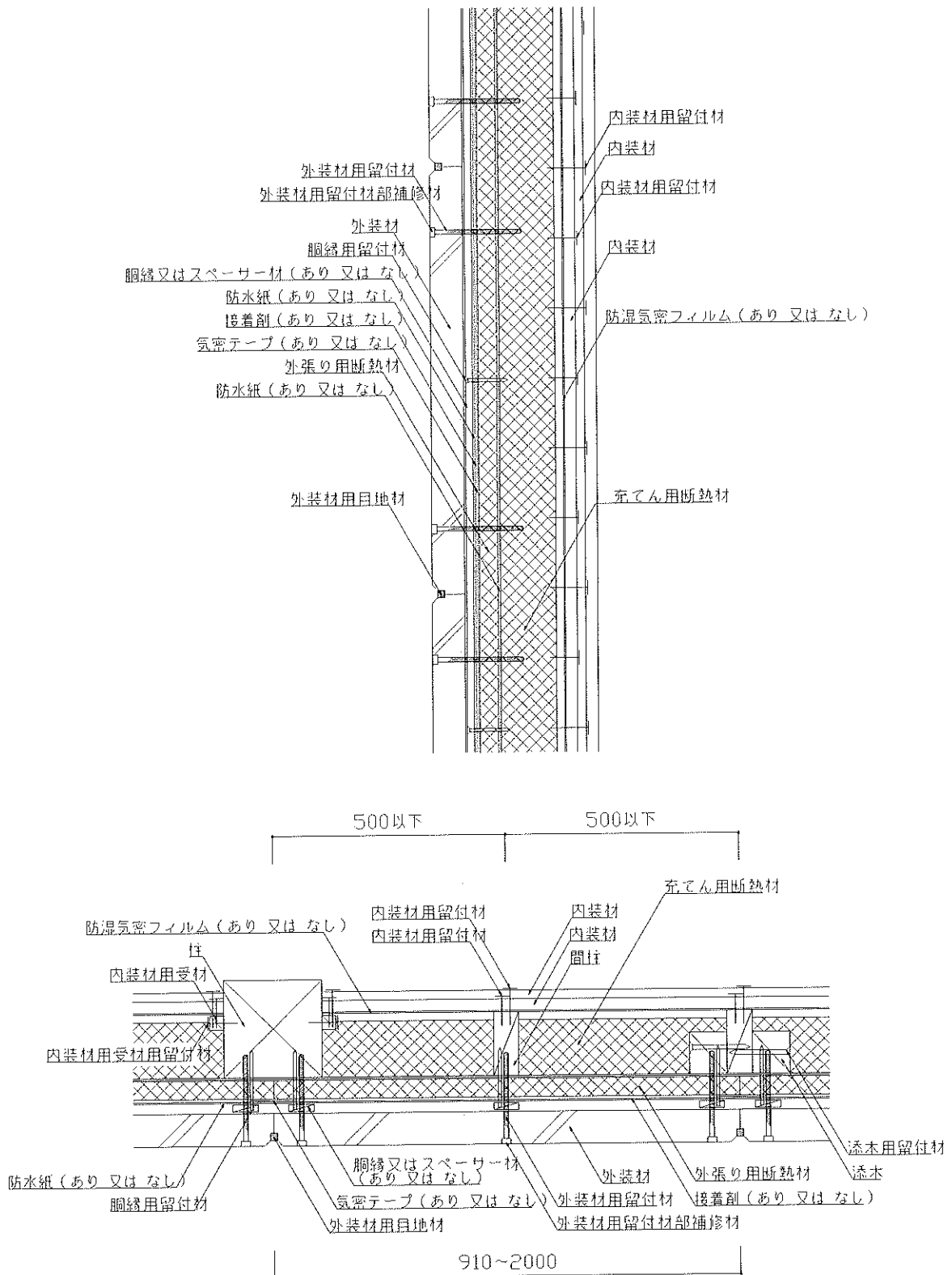
図4 構造説明図 (断面図・構造用面材なし/内装材真壁(重張②))
