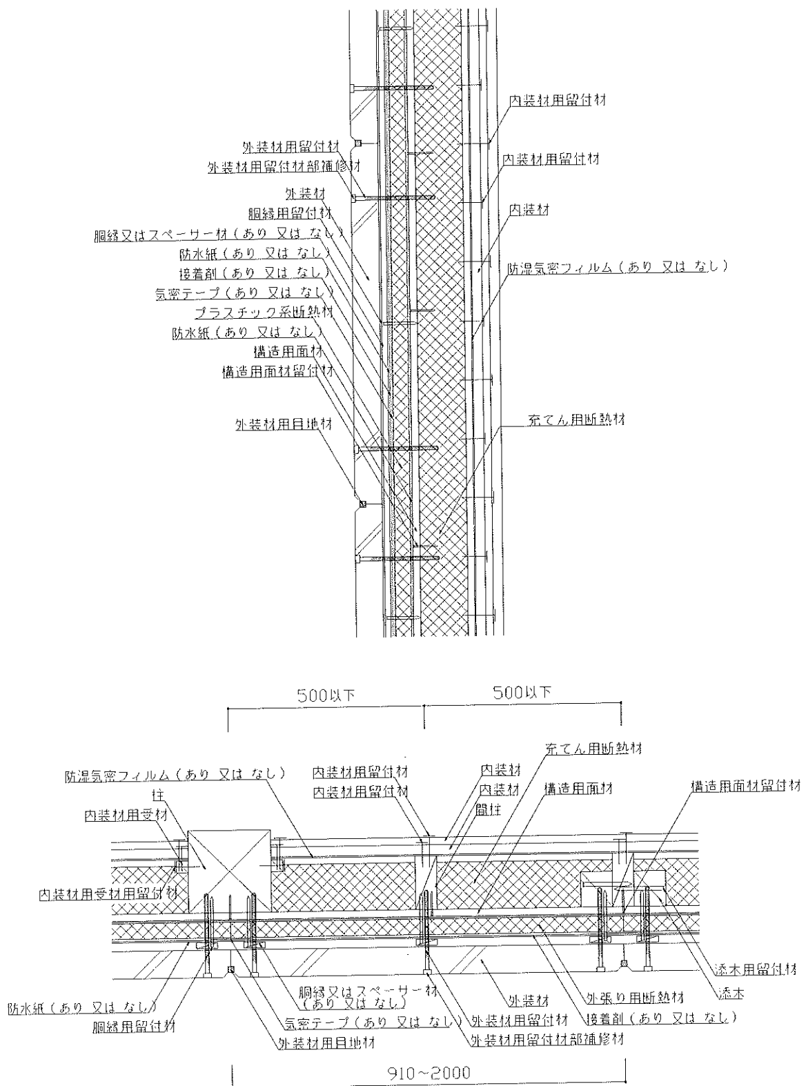
図4 構造説明図 (断面図・構造用面材大壁／内装材真壁(重張))
