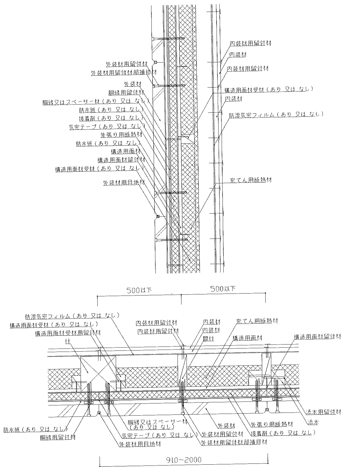
図6 構造説明図 (断面図・構造用面材真壁／内装材大壁(重張))
