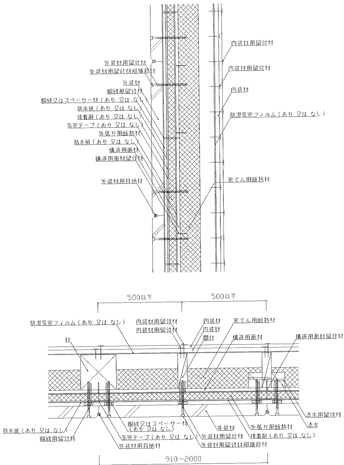
図2 構造説明図 (断面図・構造用面材大壁/内装材大壁(重張))
