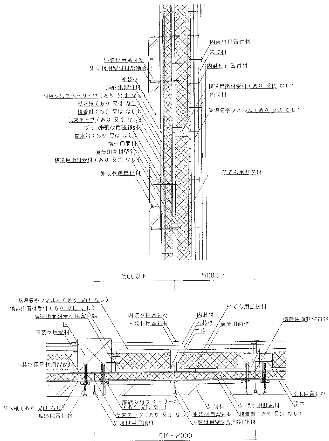
図8 構造説明図 (断面図・構造用面材真壁／内装材真壁(重張))
