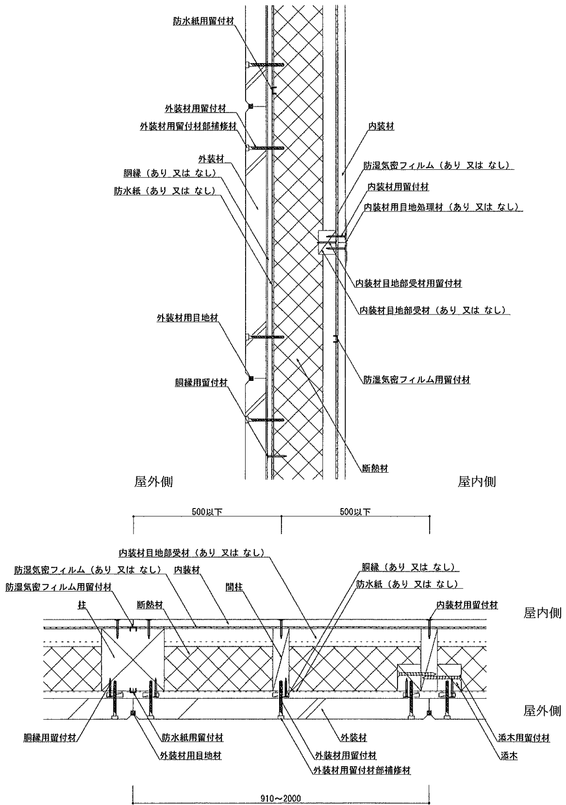
図2 構造説明図 (水平垂直断面詳細図・構造用面材なし)
