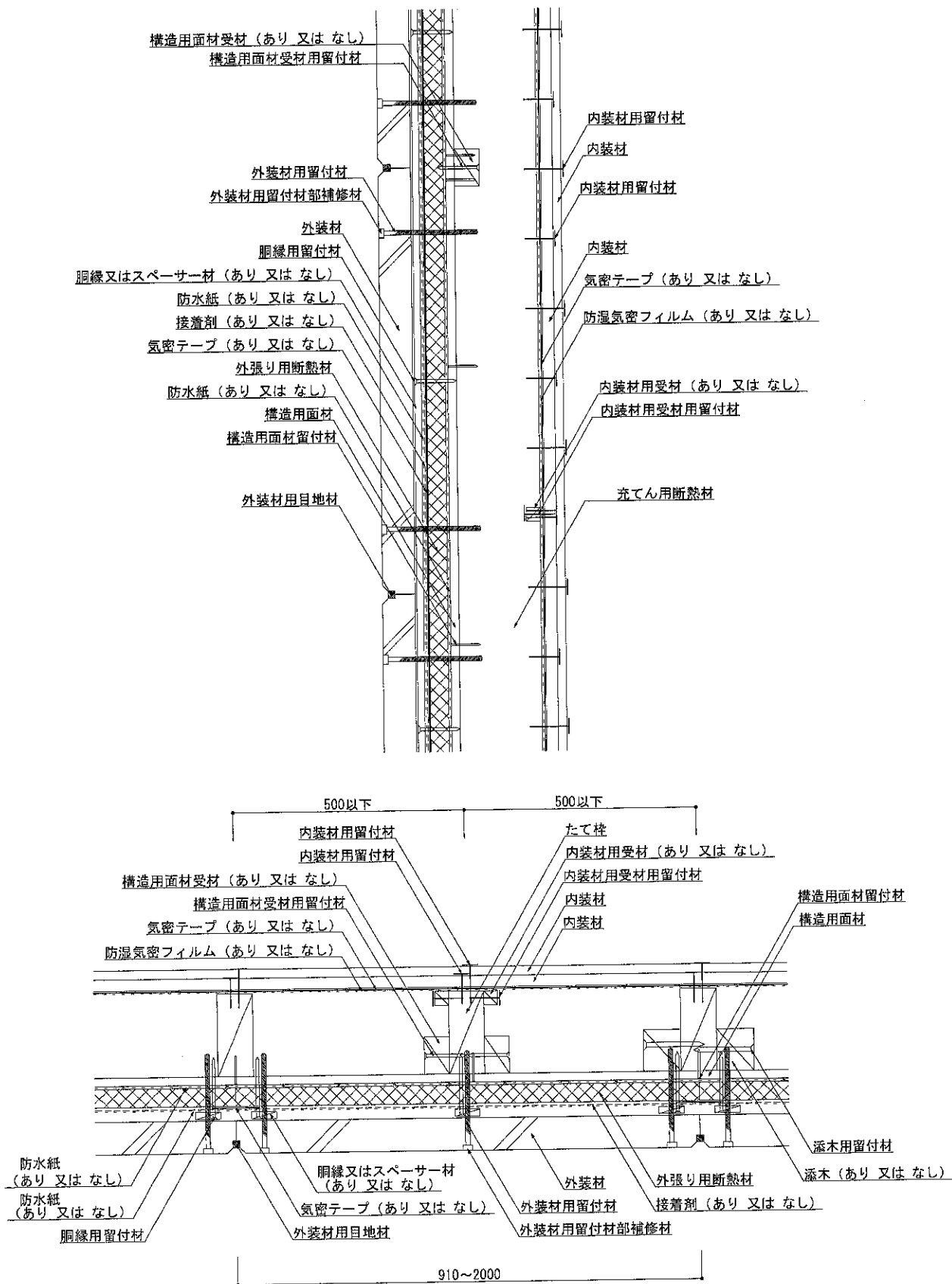
図2 構造説明図(断面図・充てん用断熱材なし／内装材重張り)
