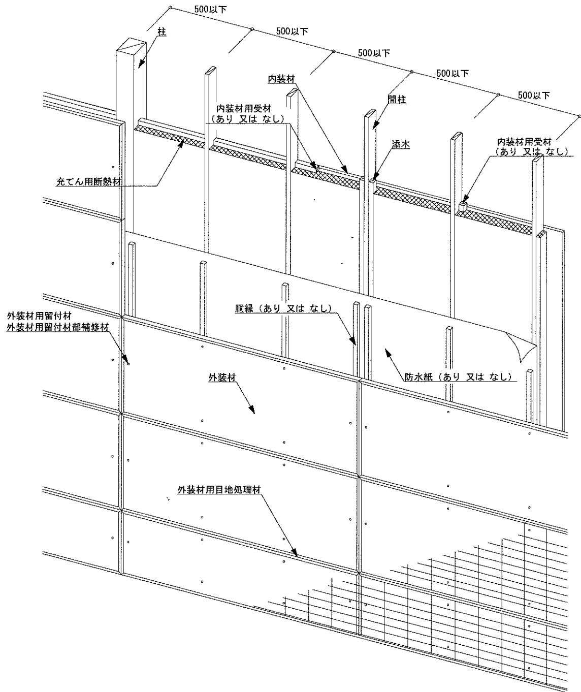
図5 構造説明図 (透視図・構造用面材なし／内装材真壁②(単張り))
