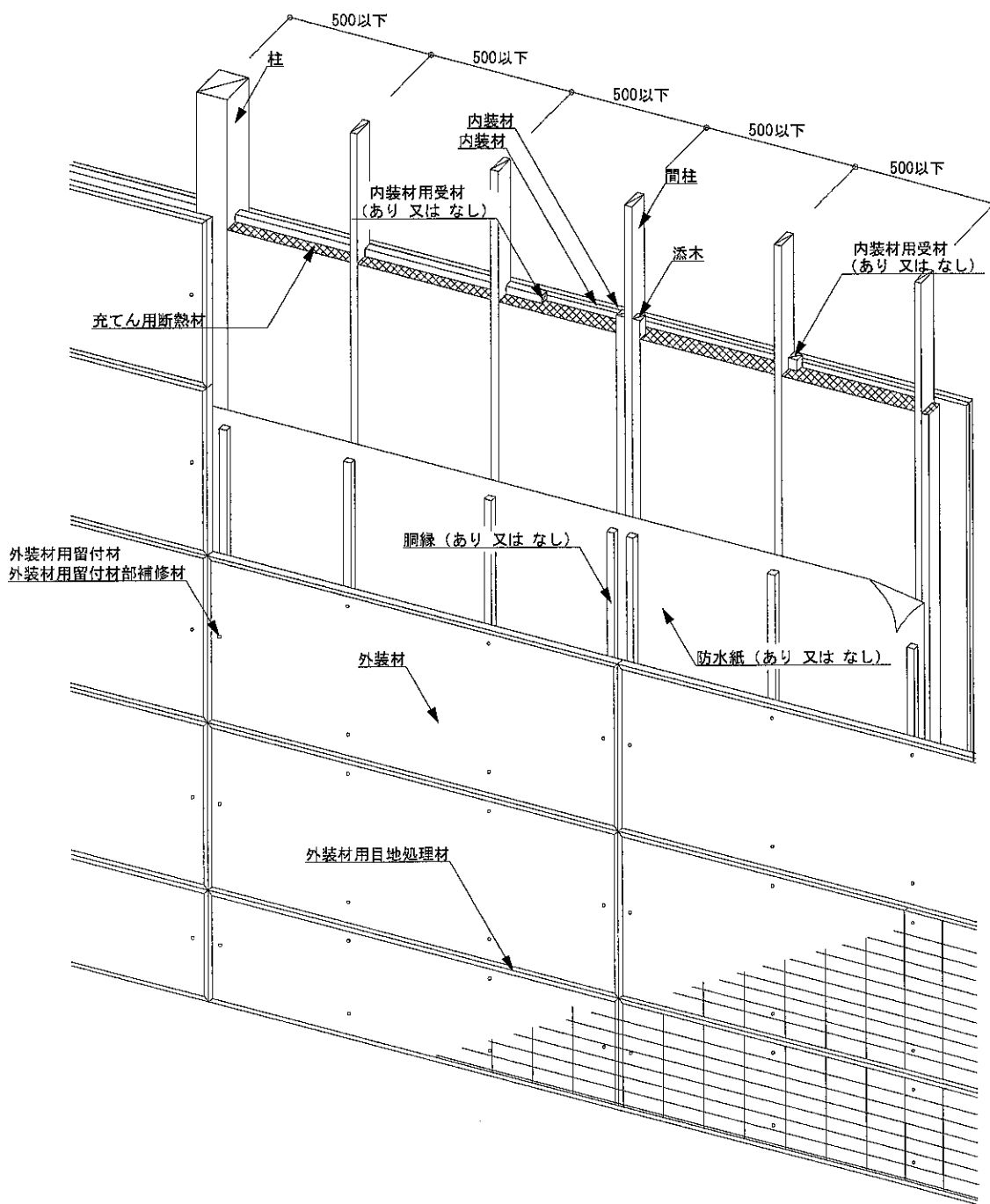
図3 構造説明図 (透視図・構造用面材なし／内装材真壁② (重張り))
