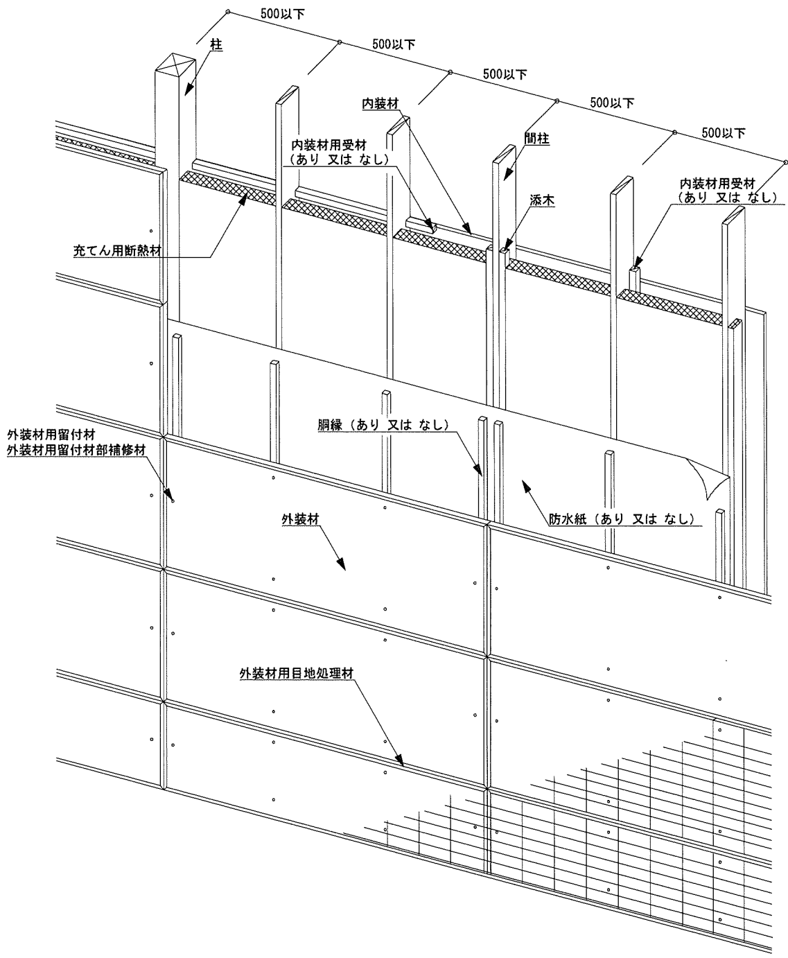
図1 構造説明図 (透視図・構造用面材なし)
