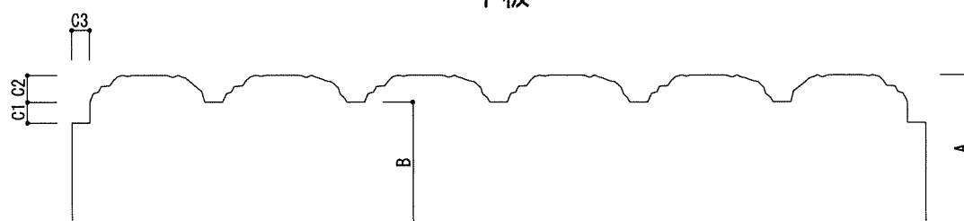
エンボス板
