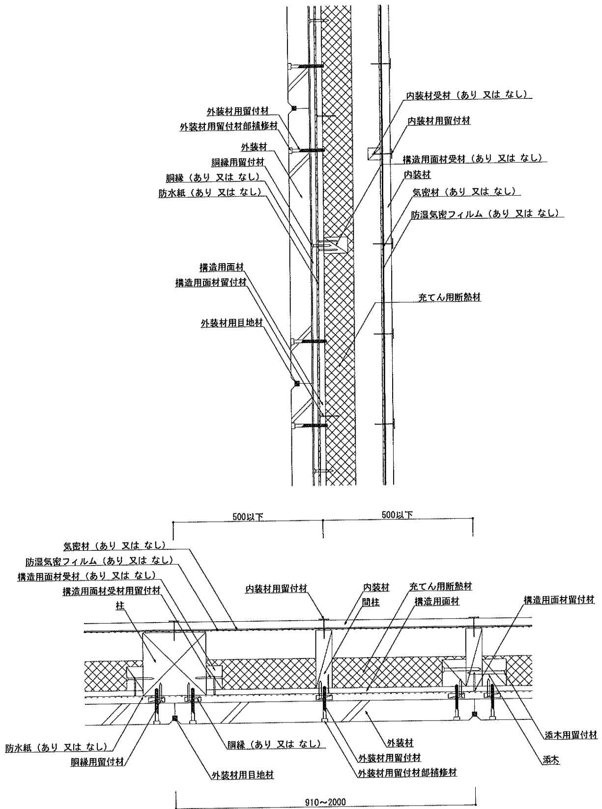
図4 構造説明図
