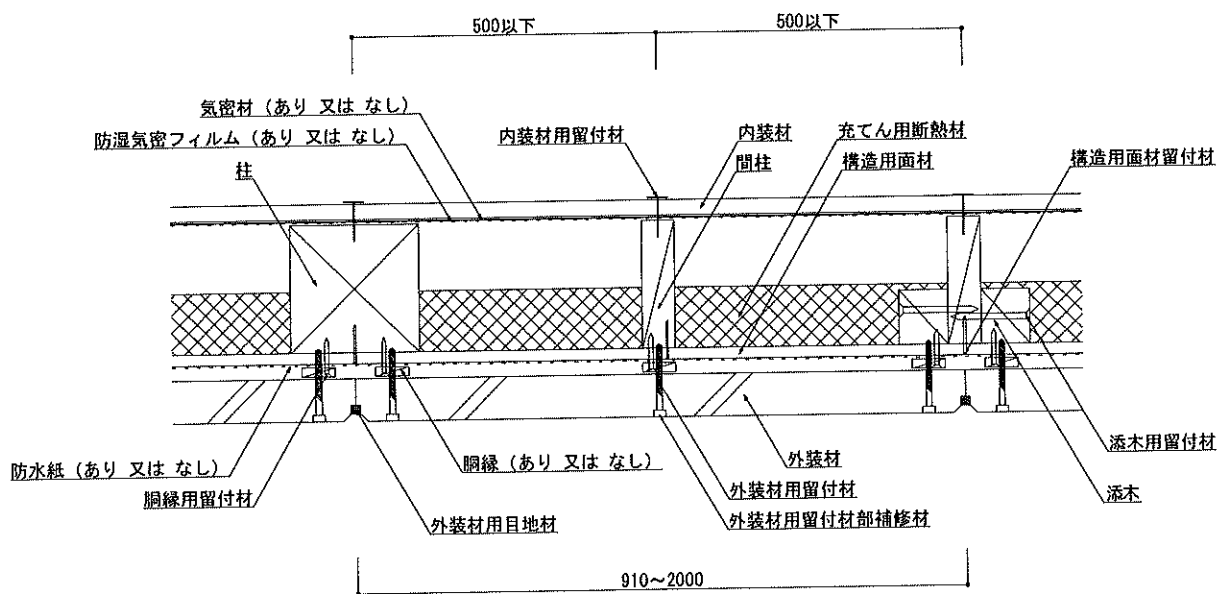
図2 構造説明図
