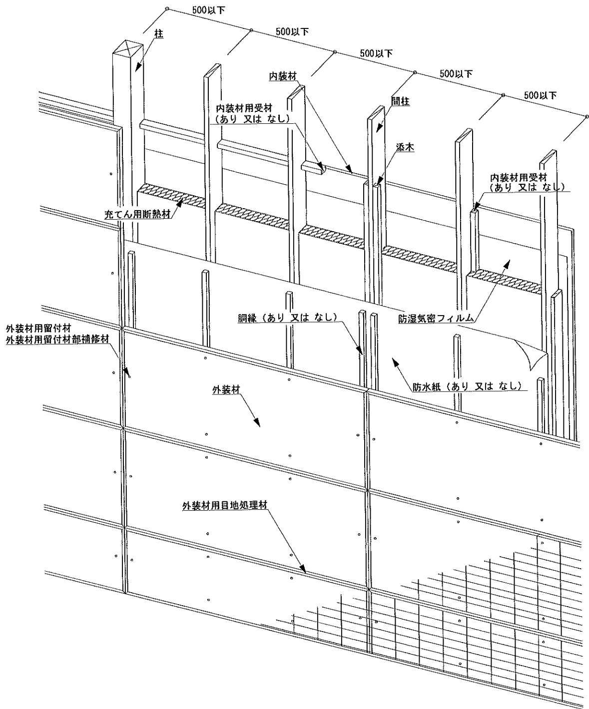
図1 構造説明図 (透視図／構造用面材なし・内装材単張・充てん断熱材あり)
