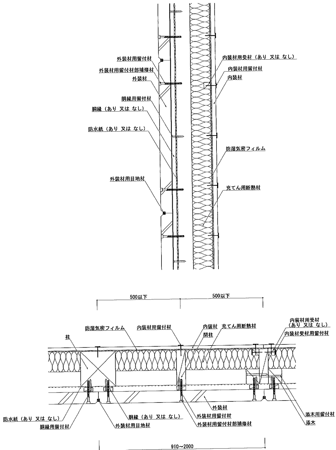
図2 構造説明図 (断面図/構造用面材なし・内装材単張・充てん断熱材あり)
