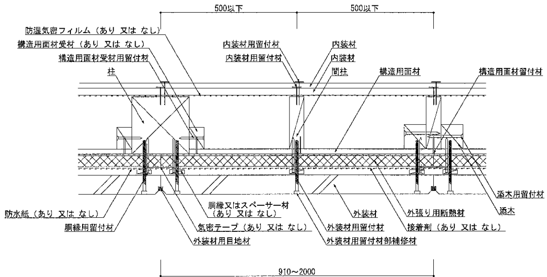
図4 構造説明図 (断面図・構造用面材真壁/内装材(重張)/充てん用断熱材なし)
