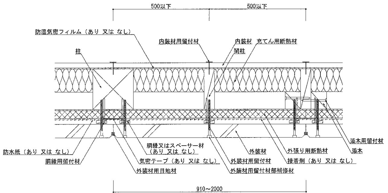
図2 構造説明図 (断面図・構造用面材なし/内装材(単張)/充てん用断熱材あり)
