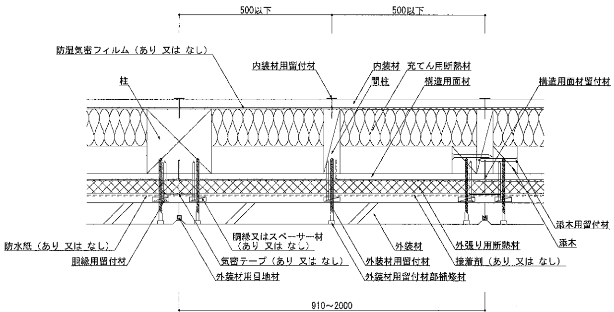
図2 構造説明図 (断面図・構造用面材大壁/内装材 (単張) /充てん用断熱材あり)
