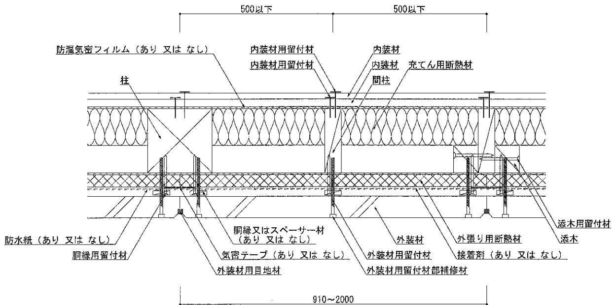
図2 構造説明図 (断面図・構造用面材なし／内装材 (重張) ／充てん用断熱材あり)
