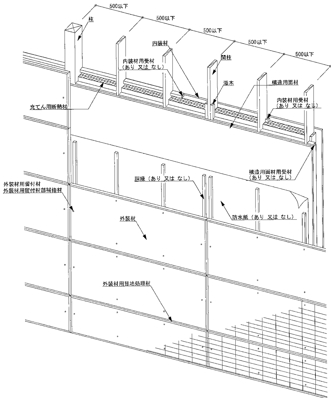
図1 構造説明図（透視図・構造用面材大壁／内装材（単張）／充てん用断熱材あり）
