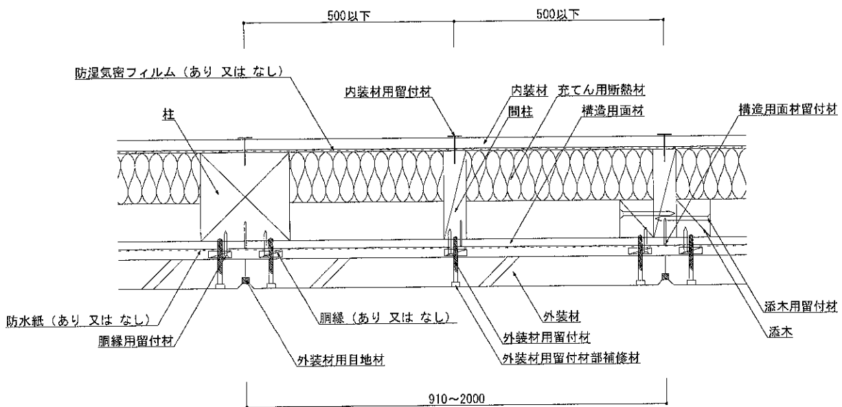
図2 構造説明図（断面図・構造用面材大壁／内装材（単張）／充てん用断熱材あり）
