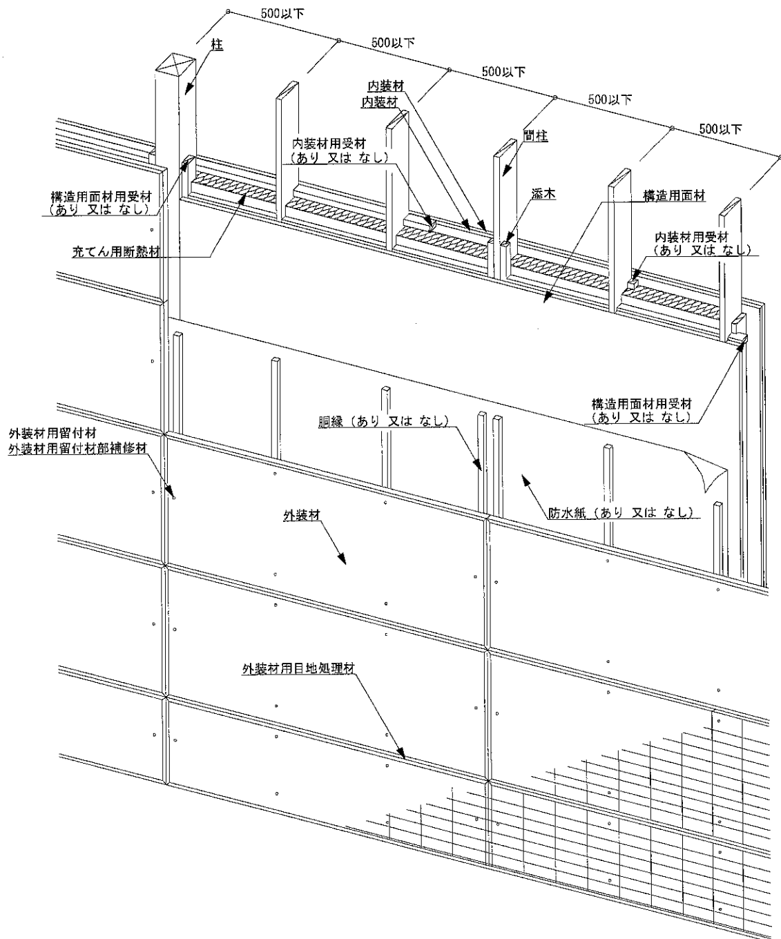
図3 構造説明図（透視図・構造用面材真壁／内装材（重張）／充てん用断熱材あり）
