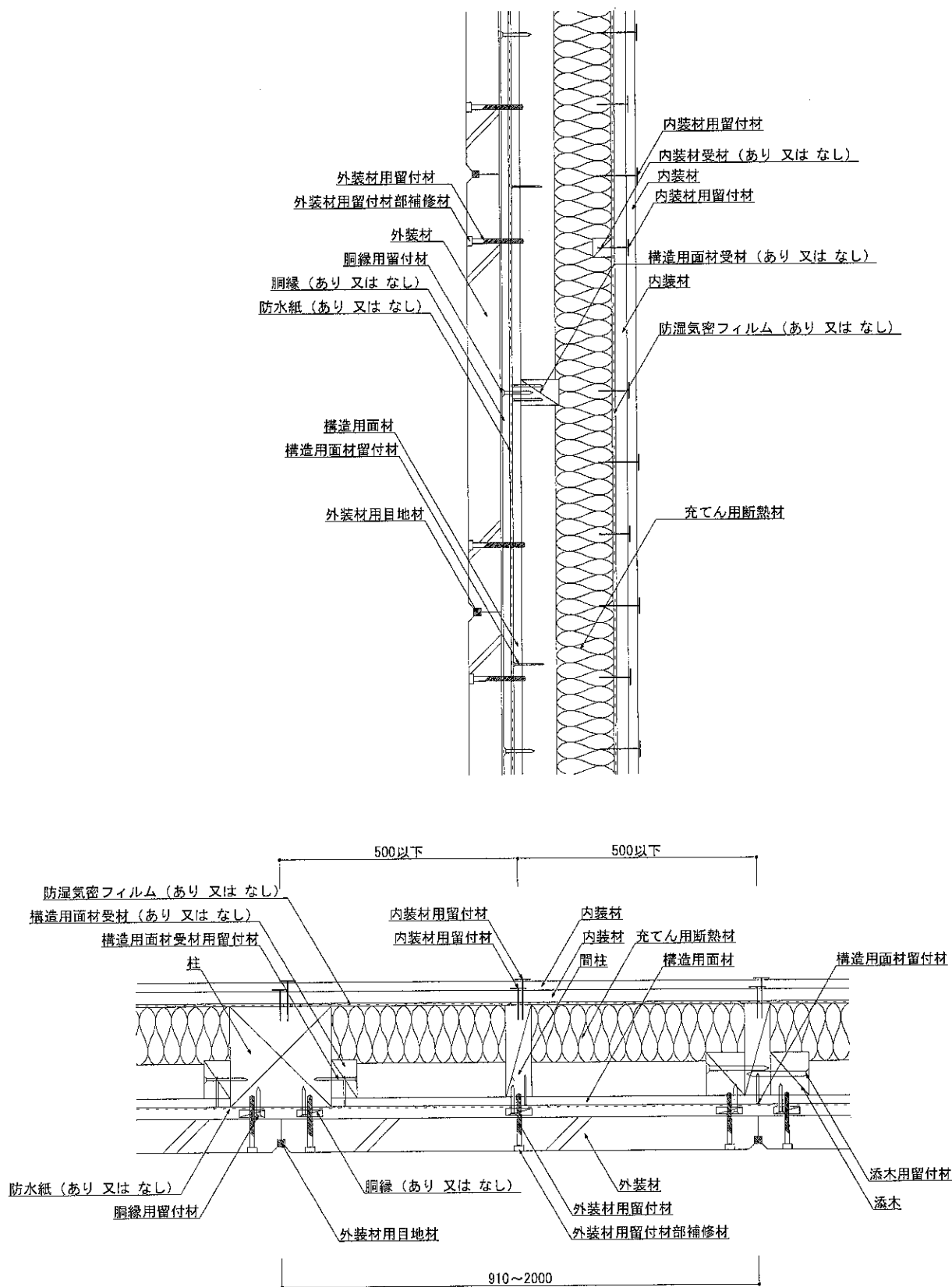
図4 構造説明図 (断面図・構造用面材真壁/内装材 (重張) /充てん用断熱材あり)
