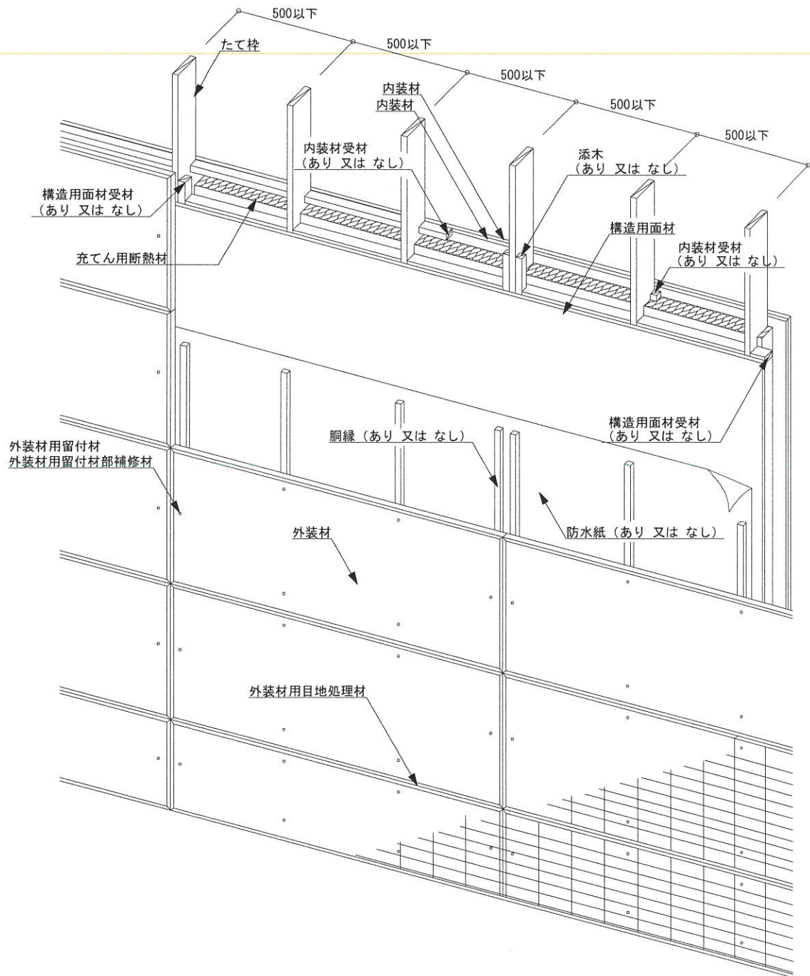
図1 構造説明図（透視図・内装材（重張））
