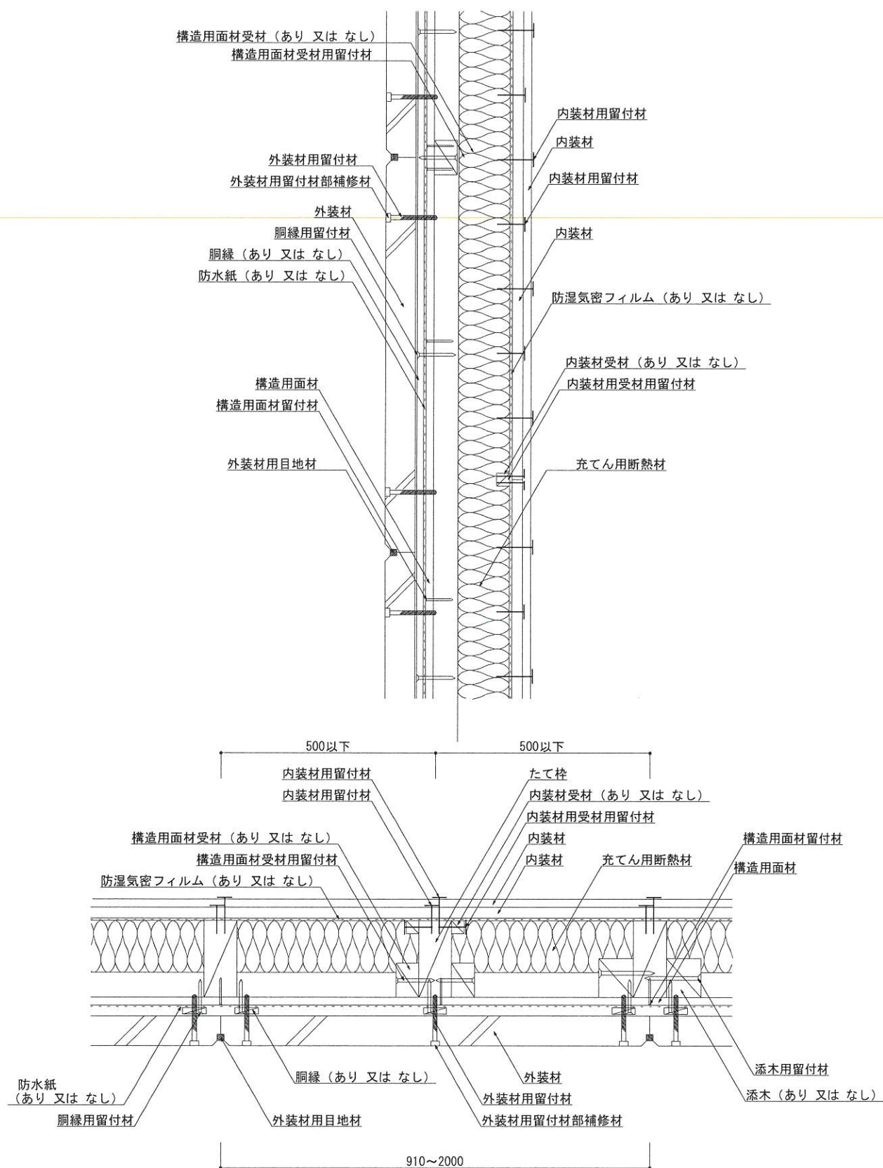
図2 構造説明図 (内装材 (重張))
