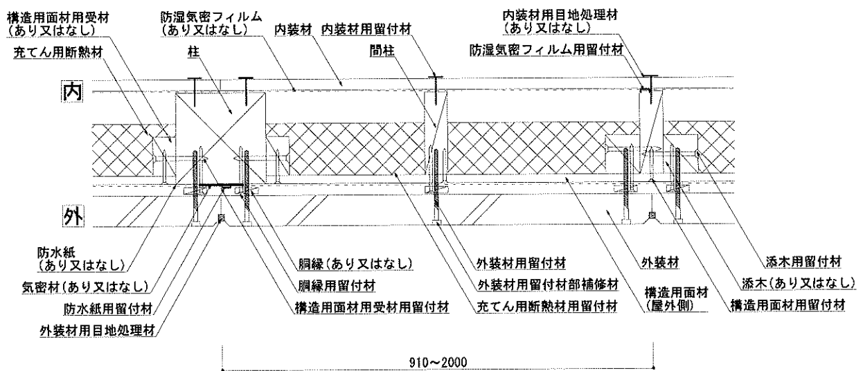
図2 構造説明図(水平垂直断面詳細図：構造用面材 屋外側真壁／屋内側なし 内装材単張仕様)
