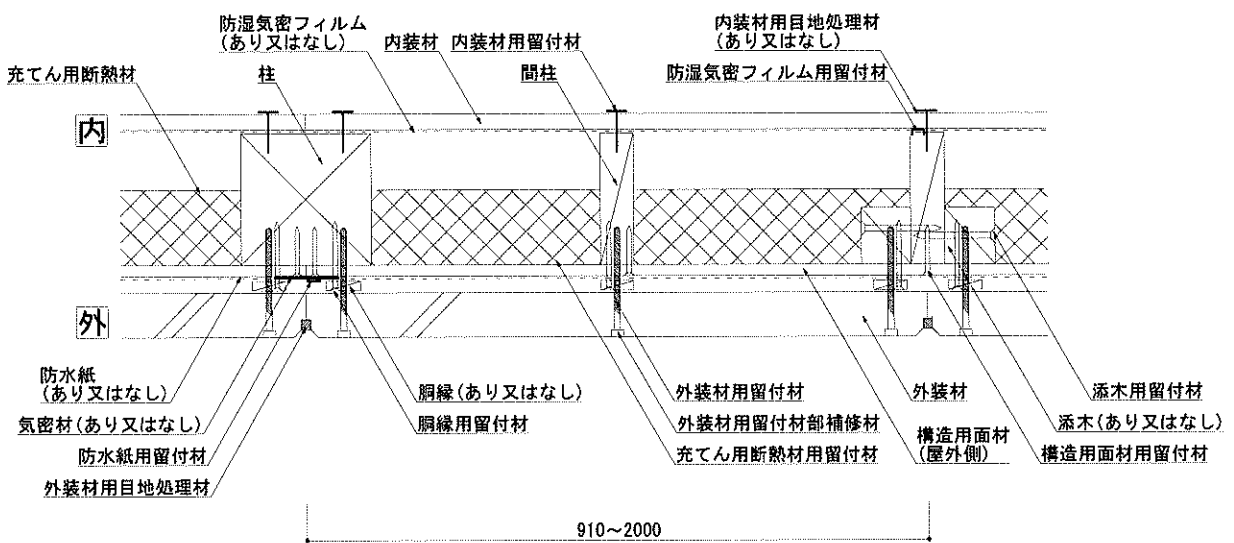
図4 構造説明図(水平垂直断面詳細図：構造用面材 屋外側大壁/屋内側なし 内装材単張仕様)
