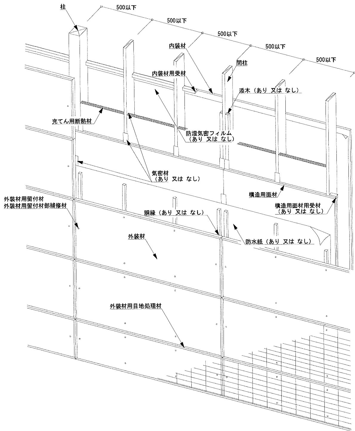
図3 構造説明図(透視図：構造用面材 屋外側大壁／屋内側なし 内装材単張仕様)
