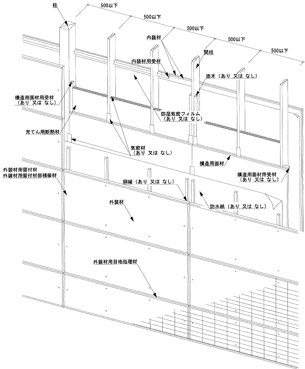
図1 構造説明図(水平垂直断面詳細図：構造用面材 屋外側真壁／屋内側なし 内装材重張仕様)
