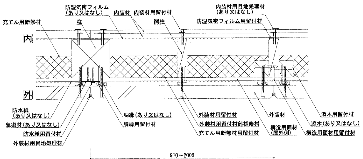
図4 構造説明図(水平垂直断面詳細図：構造用面材 屋外側大壁／屋内側なし 内装材重張仕様)
