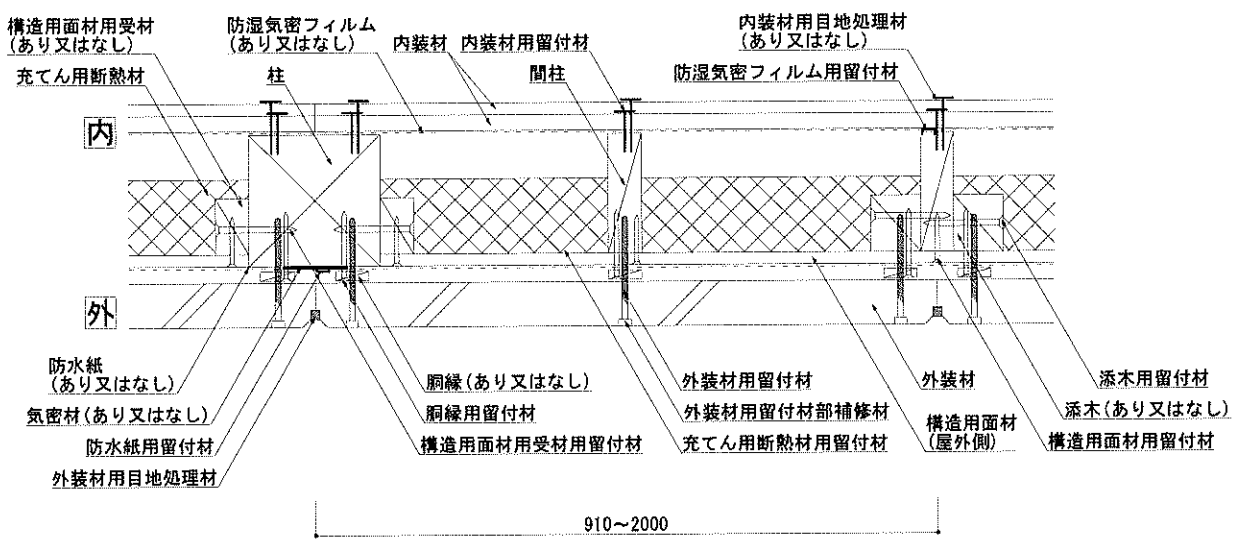
図2 構造説明図(水平垂直断面詳細図：構造用面材 屋外側真壁／屋内側なし 内装材重張仕様)
