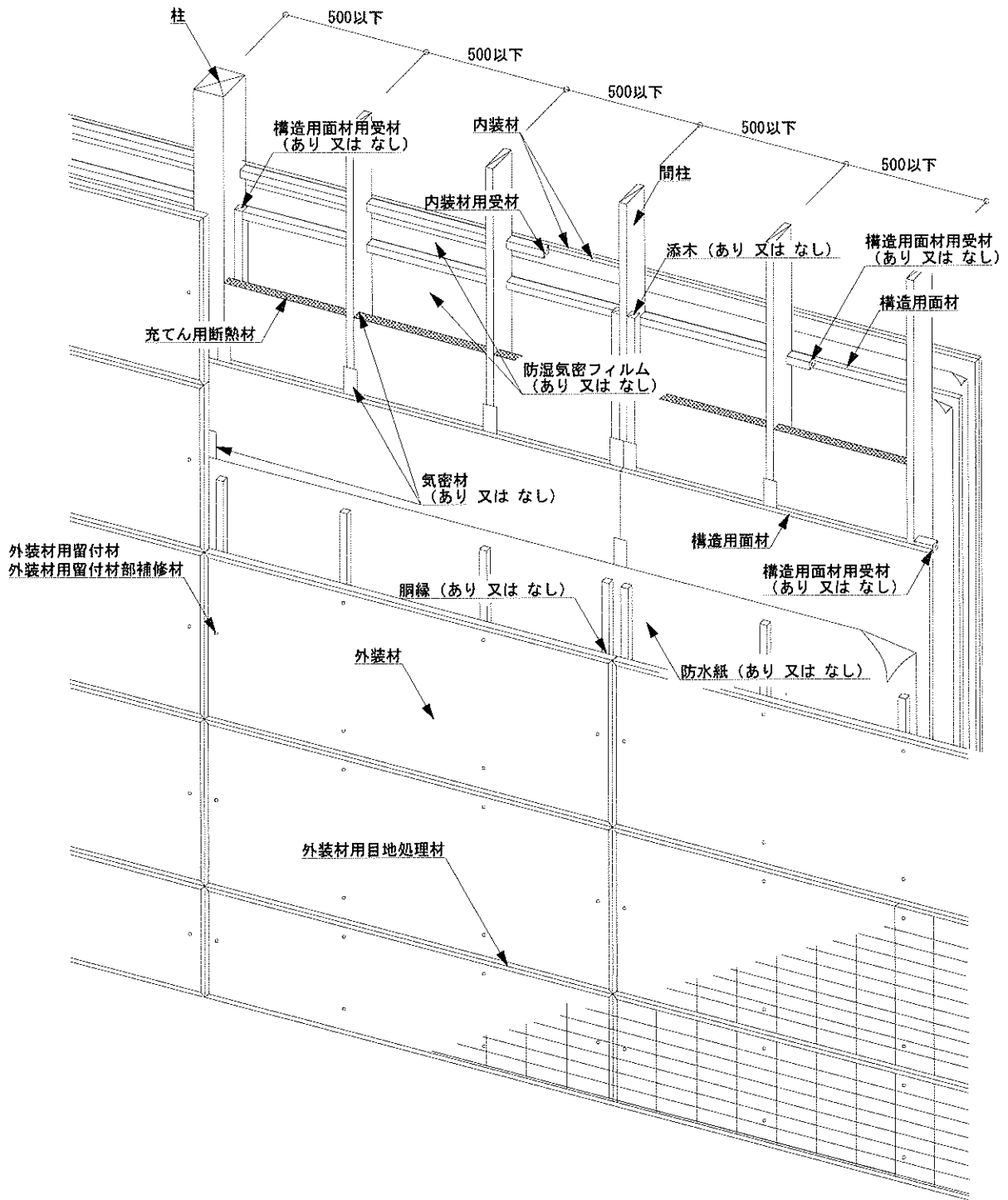
図5 構造説明図(透視図：構造用面材 屋外側大壁／屋内側真壁 内装材重張仕様)
