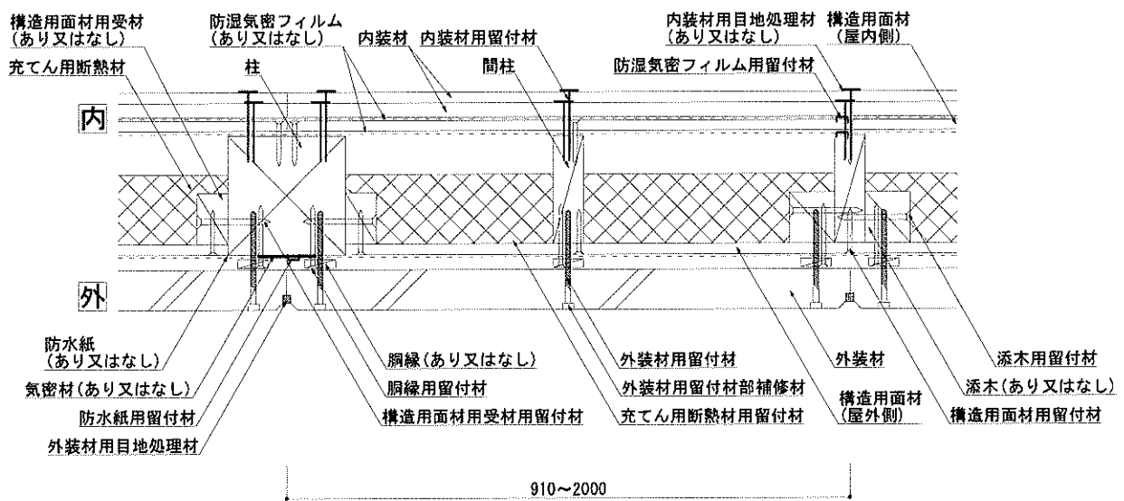
図4 構造説明図(水平垂直断面詳細図：構造用面材 屋外側真壁／屋内側大壁 内装材重張仕様)
