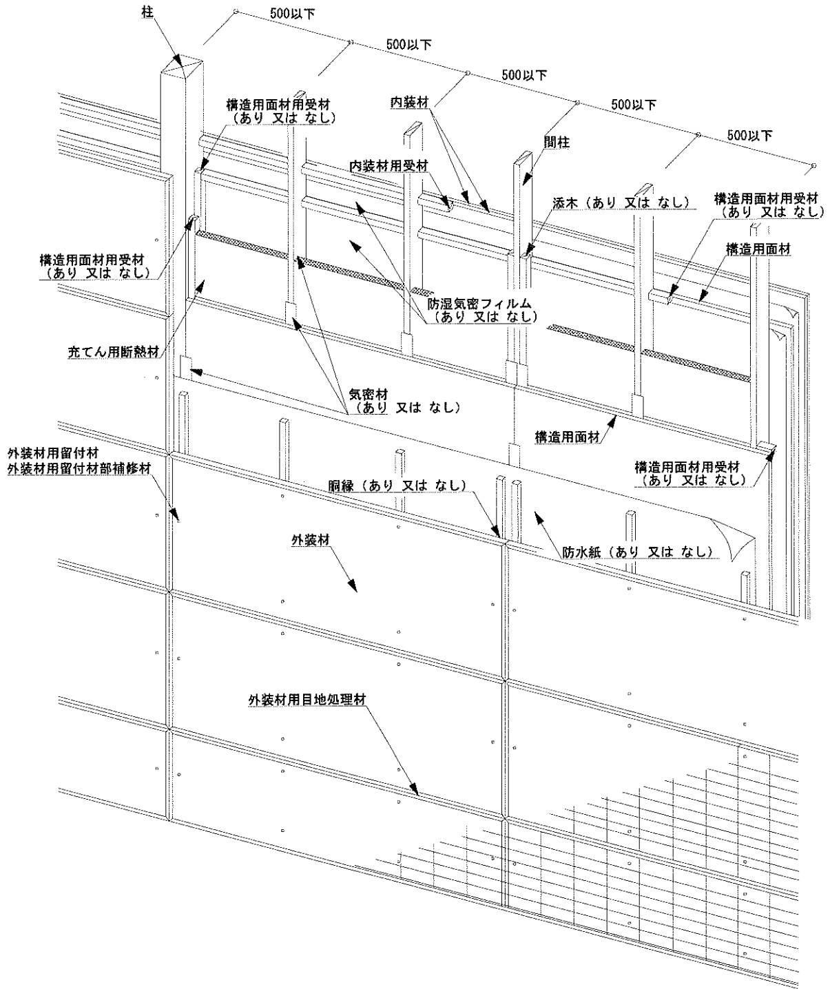
図1 構造説明図(透視図：構造用面材 屋外側真壁/屋内側真壁 内装材重張仕様)
