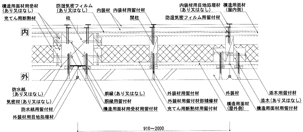
図2 構造説明図 (水平垂直断面詳細図：構造用面材 屋外側真壁/屋内側真壁 内装材重張仕様)
