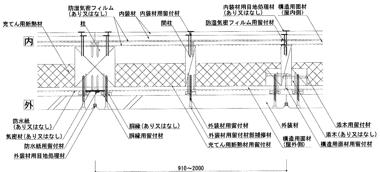
図8 構造説明図(水平垂直断面詳細図：構造用面材 屋外側大壁／屋内側大壁 内装材重張仕様)
