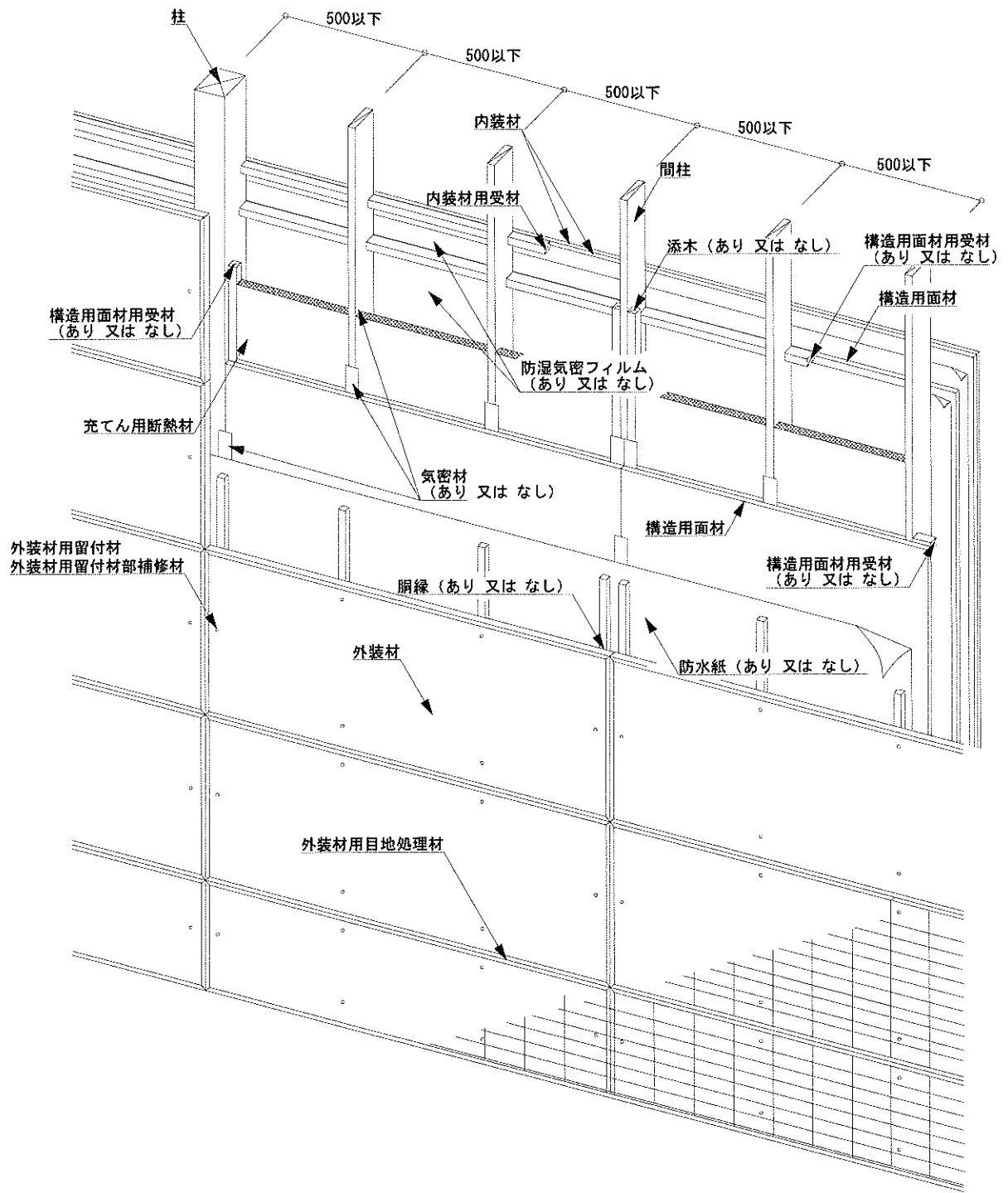
図3 構造説明図(透視図：構造用面材 屋外側真壁／屋内側大壁 内装材重張仕様)
