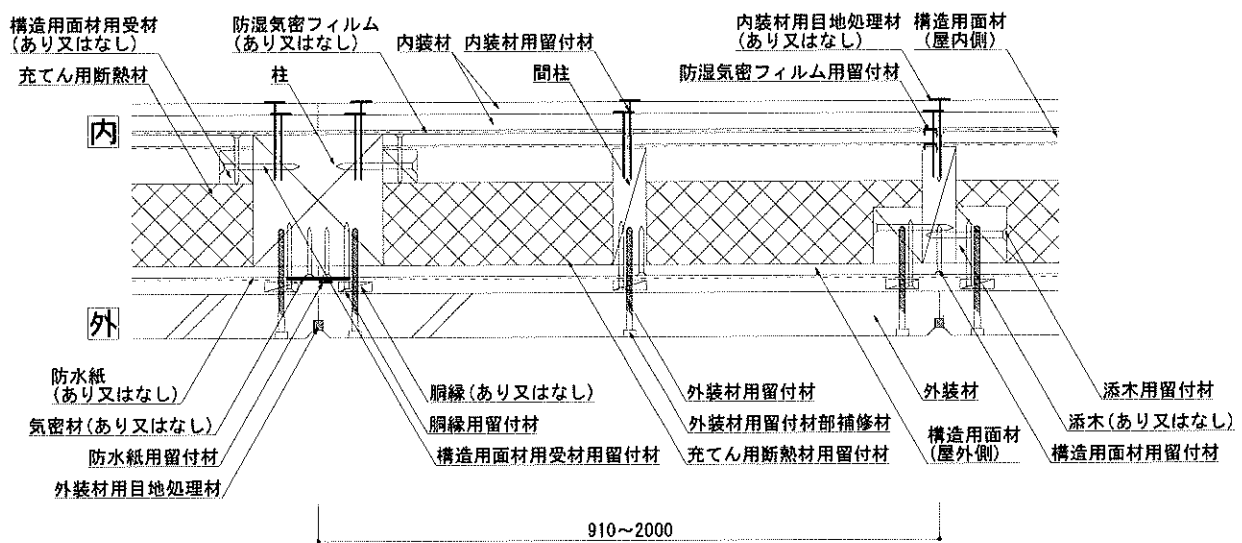
図6 構造説明図(水平垂直断面詳細図：構造用面材 屋外側大壁／屋内側真壁 内装材重張仕様)
