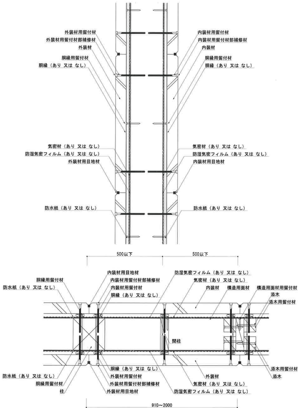
図2 構造説明図 (水平垂直断面詳細図・構造用面材なし)
