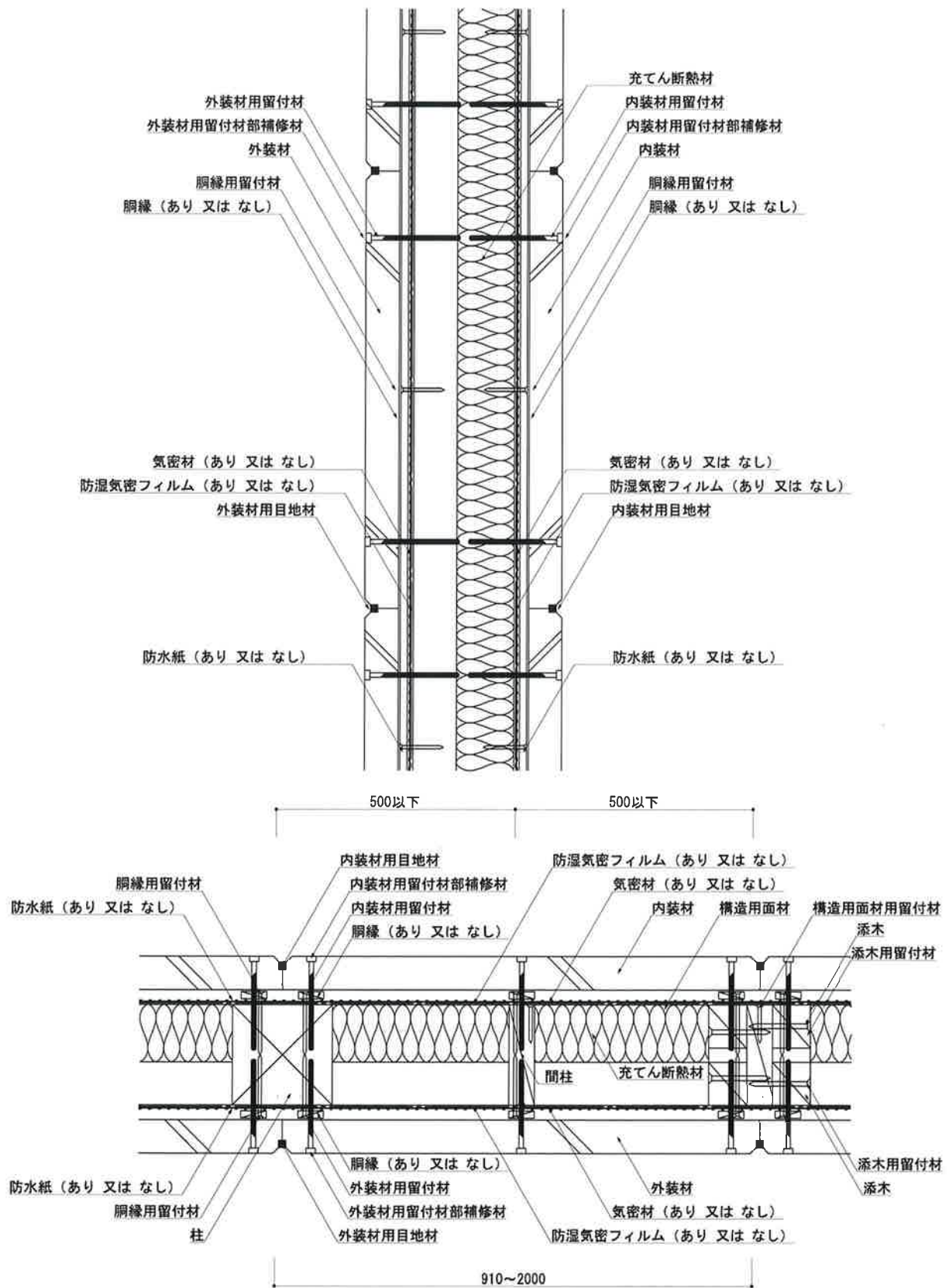
図2 構造説明図 (水平垂直断面詳細図・人造鉱物繊維断熱材充填/構造用面材なし)
