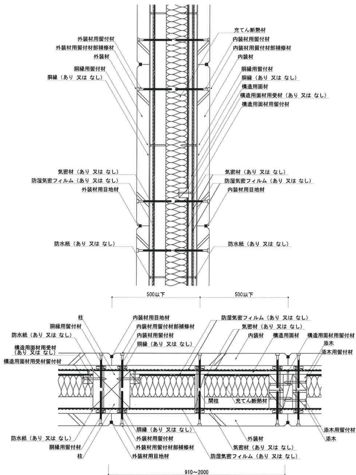
図4 構造説明図
